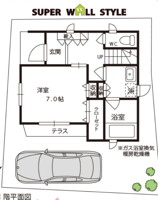
1階平面図
